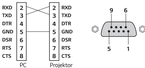
Abbildung 1: RS-232-Verbindungsdiagramm
